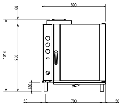
Zij aanzicht
